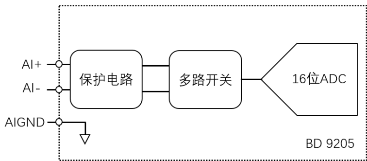
BD 9205 某通道的电路示意图
